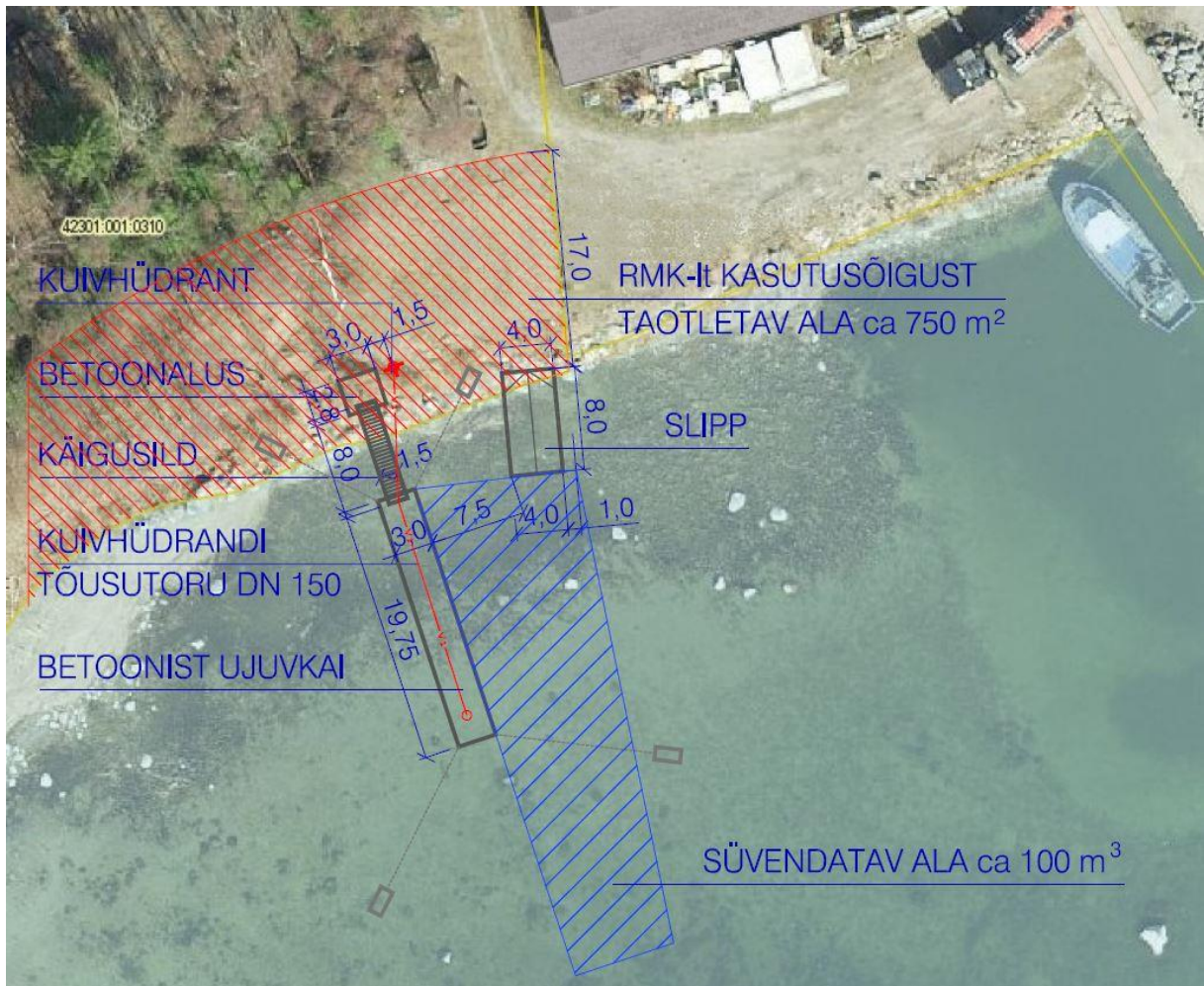
Joonis 1. Tapurla kuivhüdrandi joonis
